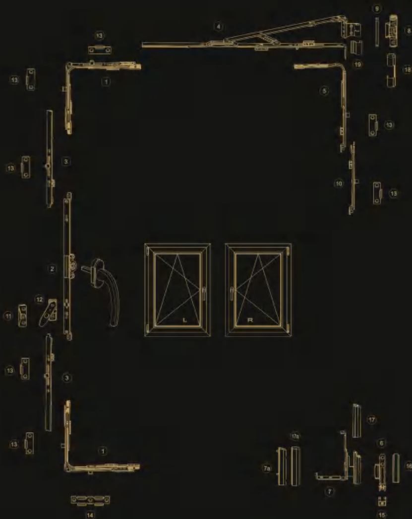
内平开/内倒五金，E5系统 Bandseite E5, Systeme 12/18 -9
